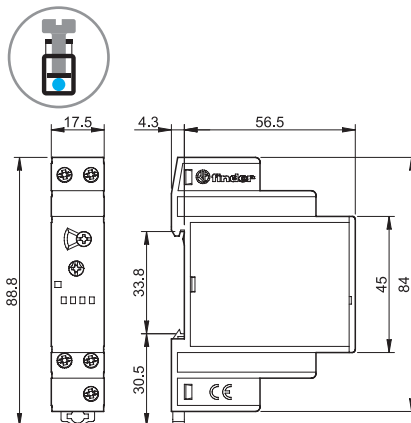
80.91 Bornes à cage
