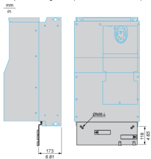
Plaque de montage CEM (fournie avec le variateur)
