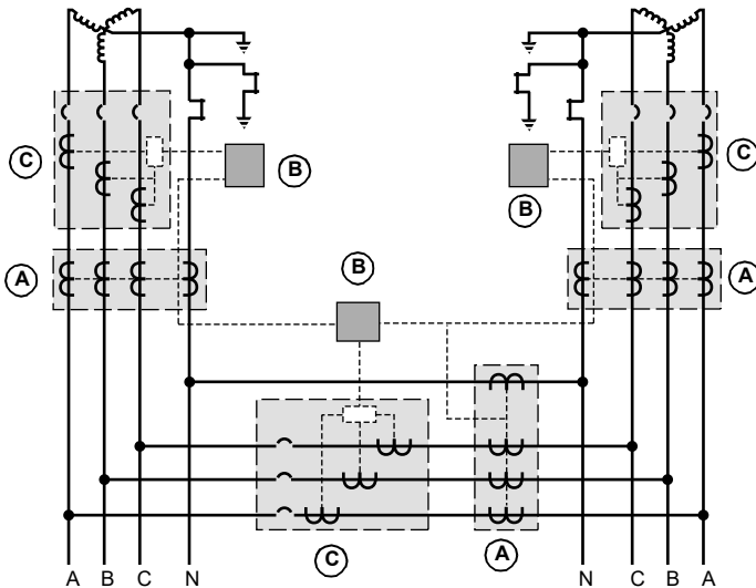
Typical Main-Tie-Main System / Système typique « principal-couplage-principal » / Sistema de tipo principal-transferencia-principal típico / Typisches Main-Tie-Main-System / Sistema principale-collegamento-principale tipico / Sistema Main-Tie-Main típico / Типовая система Сеть — Межсистемная связь — Сеть / 典型的双头系统
