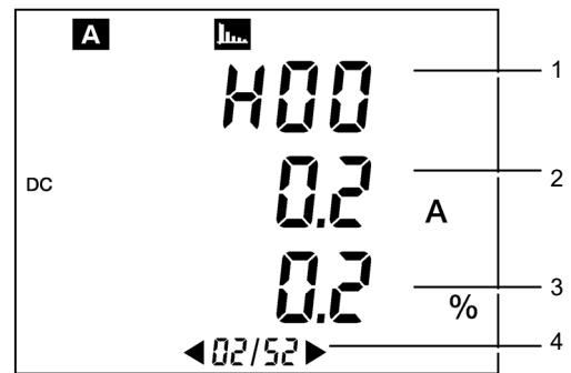
Figure 29 : Exemple d'affichage de la page 2/52.
