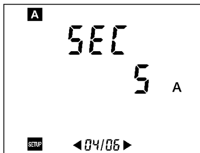
Figure 50 : Affichage du paramètre relatif au courant efficace secondaire du transformateur d'intensité.
