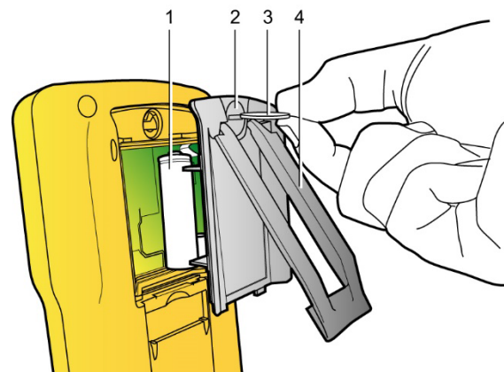
Figure 4 : Accès aux éléments de la batterie.
