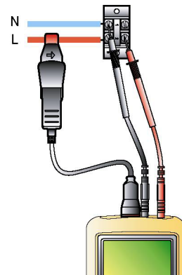
Figure 74 : Connexion en monophasé. 005
