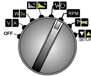
Figure 41 : Le commutateur rotatif en position RPM .
