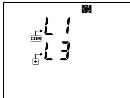
Figure 38 : Le C.A. 8220 est prêt pour la seconde mesure de détermination de l'ordre des phases.
