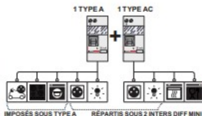
Schéma de câblage à l'intérieur
