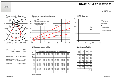
IFGU1_DN461B1xLED11S830C
