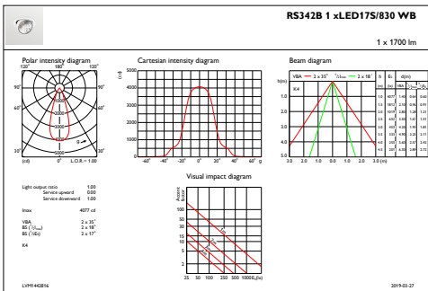
IFAS1_RS342B1xLED175S830WB
