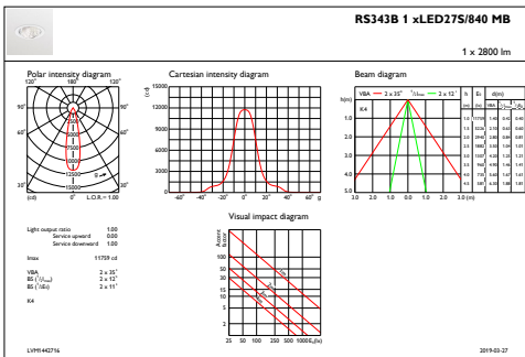
IFAS1_RS343B1xLED27S840MB
