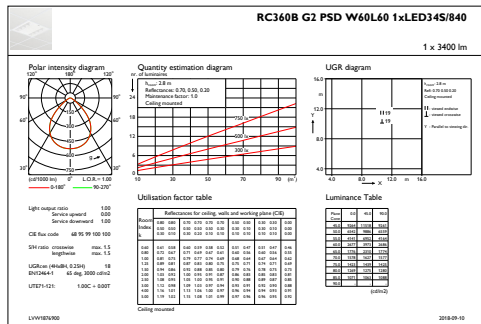
IFGU1_RC360BG2PSDW60L601xLED34S840
