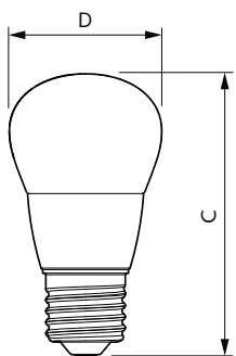
MASTER LEDlustre DT 2.8-25W E27 P48 CL
