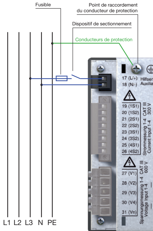
Fig. Exemple de raccordement ; raccordement de la tension d'alimentation à un UMG511.
