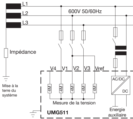
Fig. Schéma de principe, UMG511 dans réseau IT sans N.
