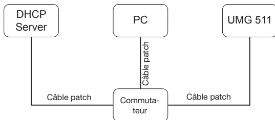
Fig. Exemple de raccordement, une adresse IP est automatiquement attribuée à l'UMG604 et au PC par un serveur DHCP.
