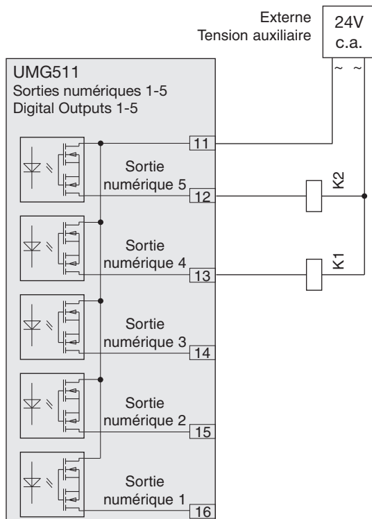
Fig. Raccordement de deux relais aux sorties numériques 4 et 5.
