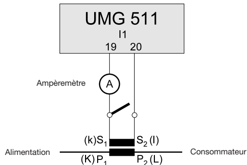
Fig. Exemple, mesure de l'intensité par un ampèremètre supplémentaire.
