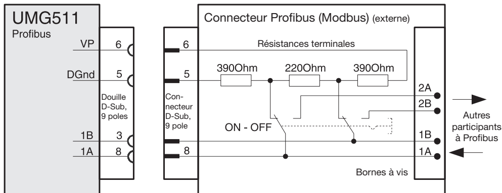
Fig. Connecteur de Profibus avec résistances de terminaison.
