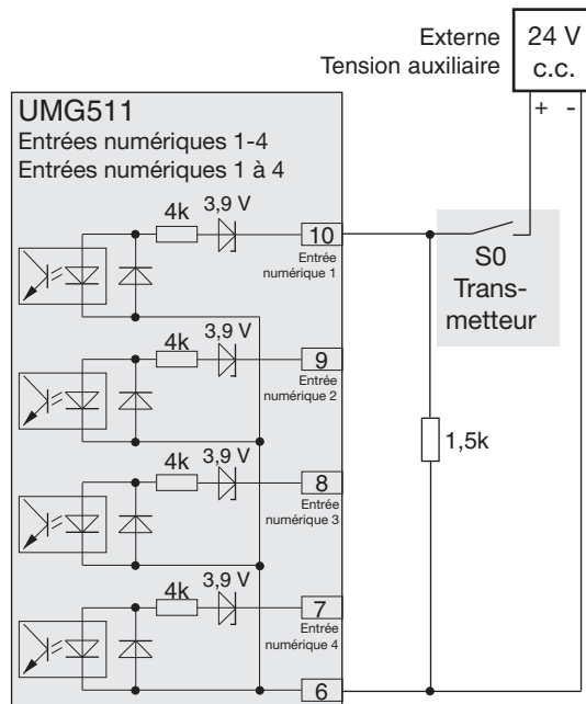
Fig. Exemple du raccordement d'un générateur d'impulsions S0 à l'entrée numérique 1.
