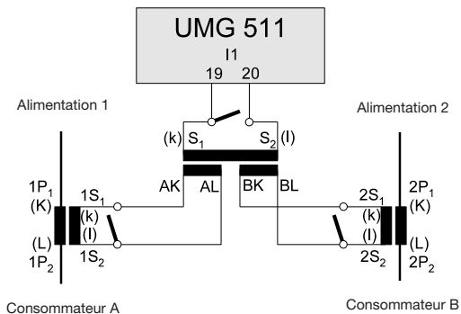
Fig. Exemple, mesure de l'intensité par un transformateur de courant sommateur.
