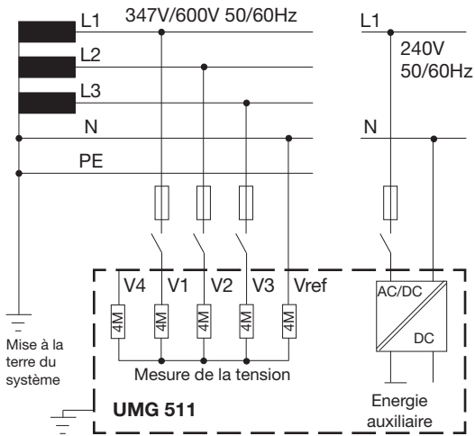
Fig. Schéma de principe, UMG511 dans le réseau TN.
