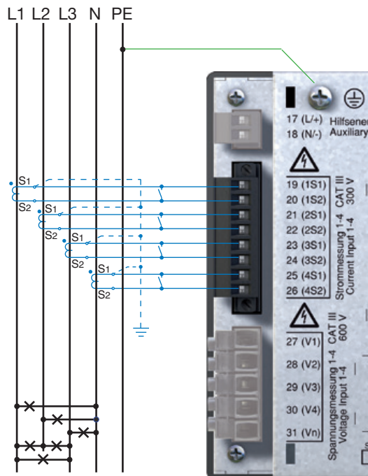
Fig. Exemple de raccordement, mesure d'intensité par transformateur d'intensité.
