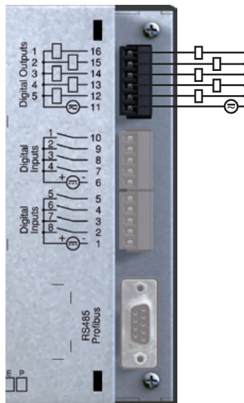
Fig. Raccordement de sorties numériques.
