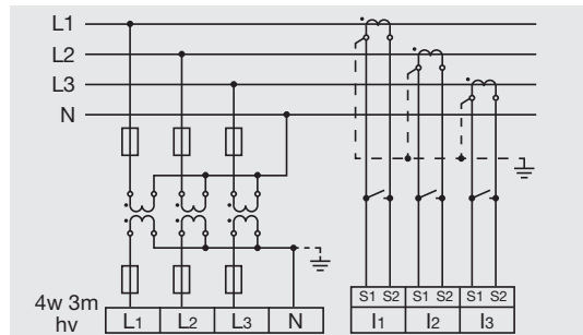
Fig. Mesure par 3 transformateurs de tension sur un réseau triphasé à 4 conducteurs à charge dissymétrique.
