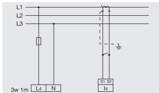
Fig. Mesure sur un réseau triphasé à 3 conducteurs à charge symétrique.
