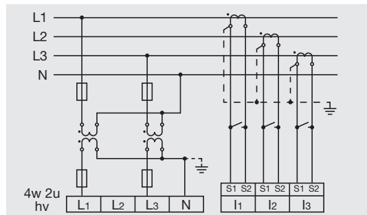
Fig. Mesure par 2 transformateurs de tension sur un réseau triphasé à 4 conducteurs à charge dissymétrique.
