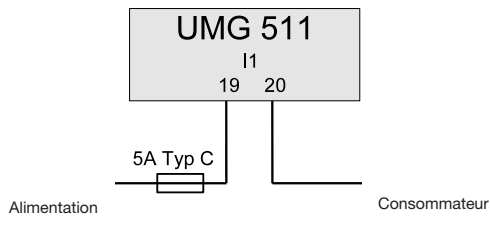
Fig. Exemple, mesure directe de la tension.
