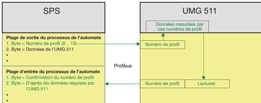
Fig. Schéma-bloc pour l'échange de données entre SPS et UMG511.
