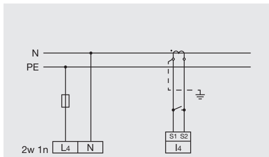
Fig. Mesure de la tension entre N et PE. Mesure du courant sur le conducteur neutre.
