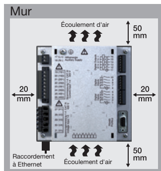
Fig. Position de montage de l'UMG511 ; vue de l'arrière.
