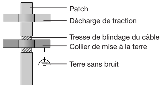
Fig. Conception du blindage à l'entrée dans l'armoire.
