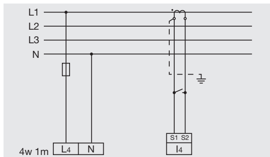
Fig. Mesure sur un réseau triphasé à 4 conducteurs à charge symétrique.
