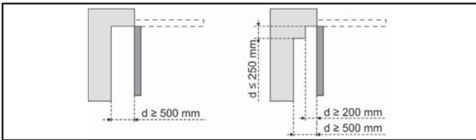
Figure 2 - Protection mécanique
