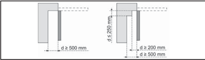
Figura 2 - Protezione meccanica
