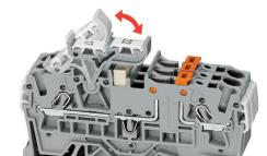
Adaptateur de marquage à deux étages pivotant (2002-121) et terminal de mesure et de déconnexion à 2 fils (2002-1671)
