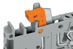
Borne sectionnable et de mesure avec couteau pivotant et avec verrouillage mécanique Sectionneur en position ouverte
