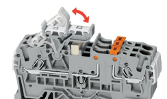
Adaptateur de marquage à deux étages pivotant (2002-121) et terminal de mesure et de déconnexion à 2 fils (2002-1671)
