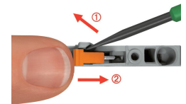
Borne sectionnable et de mesure avec couteau pivotant et avec verrouillage mécanique Fermer le sectionneur.
