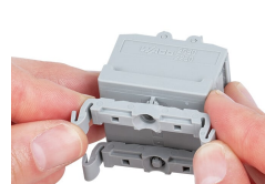
Bornier ; avec pieds de fixation à encliquer encliqueter encliqueter du pied de montage (209-120) (La distance entre les adaptateurs de montage sous la barrette à bornes doit être env. de 20 ... 25 mm.)
