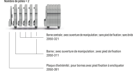
Exemple de bornettes à 5 pôles; avec ouverture de manipulation; avec pied de fixation à encliqueter Nombre de pôles = 2
