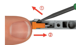
Borne sectionnable et de mesure avec couteau pivotant et avec verrouillage mécanique Fermer le sectionneur.
