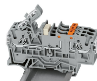
Adaptateur de marquage à deux étages pivotant (2002-121) et terminal de mesure et de déconnexion à 2 fils (2002-1671)
