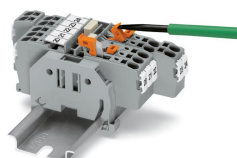
Borne sectionnable et de mesure avec support pivotant du sectionneur Ouvrir le sectionneur.
